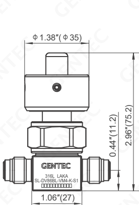
B: Handgrip (300 psi)
